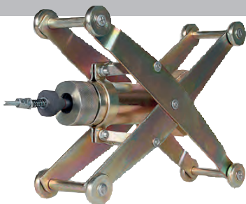
Sistema di sabbatura interna tubi da 3"(7,5 mm) a 12"(300 mm) Internal pipe blast tool 3"(7,5 mm) a 12"(300 mm)
